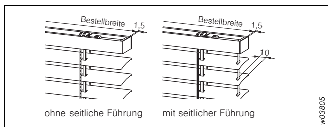
Abb. 34: Seitliche Führung
