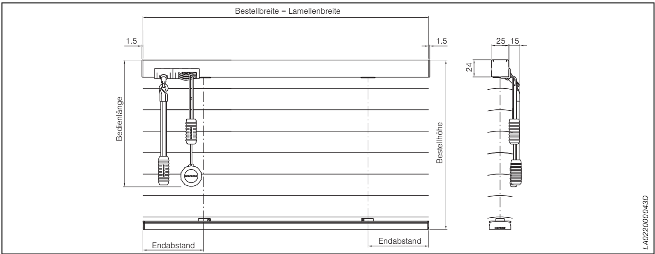
Abb. 37: Jalousie Select S – Maanleitung, Bedienung Schnur/Stab, einseitig (Standard)
