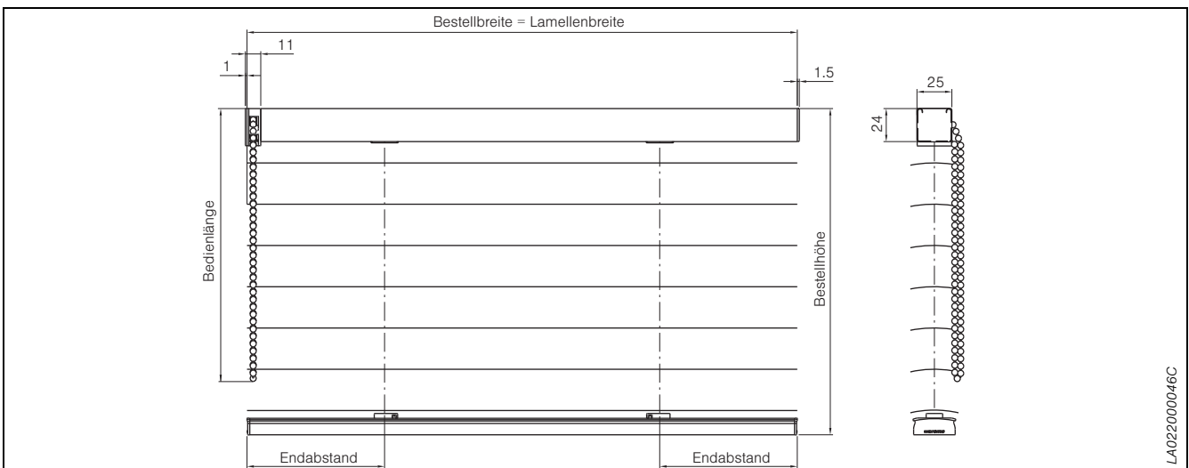
Abb. 39: Jalousie Select S – Maßanleitung, Bedienung Kugelkette
