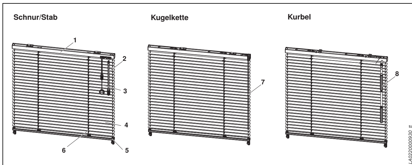
Abb. 33: Übersicht Jalousie Select S
