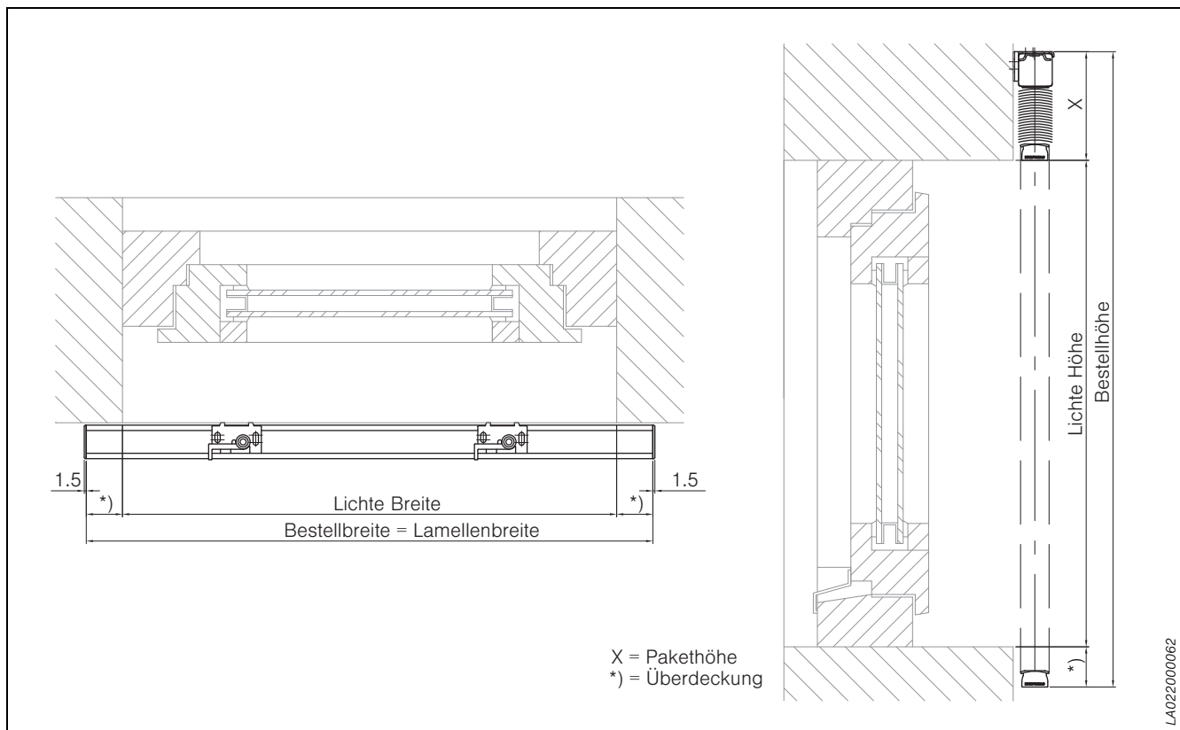
Abb. 42: Horizontal- und Vertikalschnitt – Montage vor der Laibung
