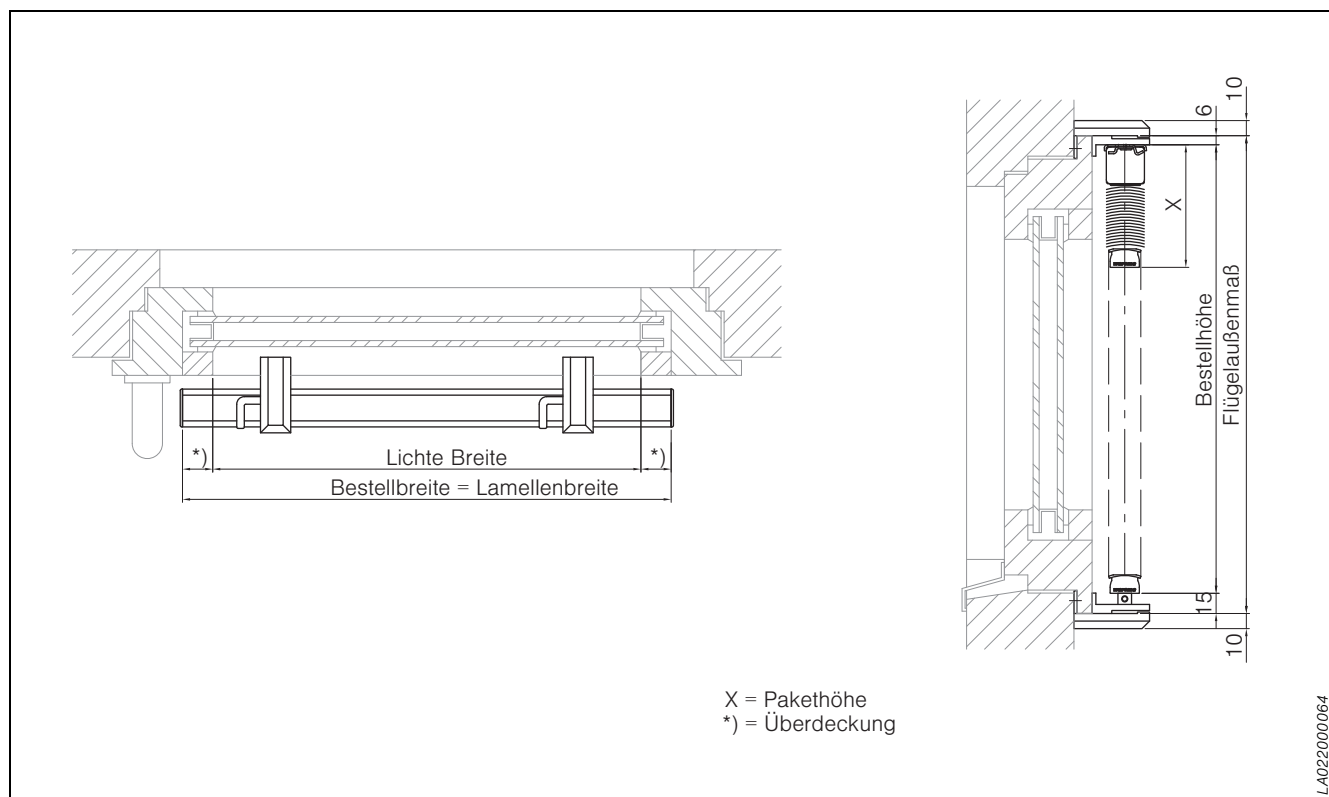
Abb. 44: Horizontal- und Vertikalschnitt – Montage mit Klemmträgern
