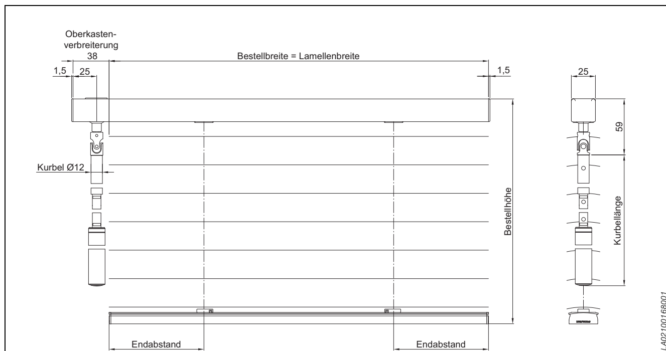
Abb. 41: Jalousie Select S – Maßanleitung, Bedienung Kurbel, Getriebeabgang senkrecht
