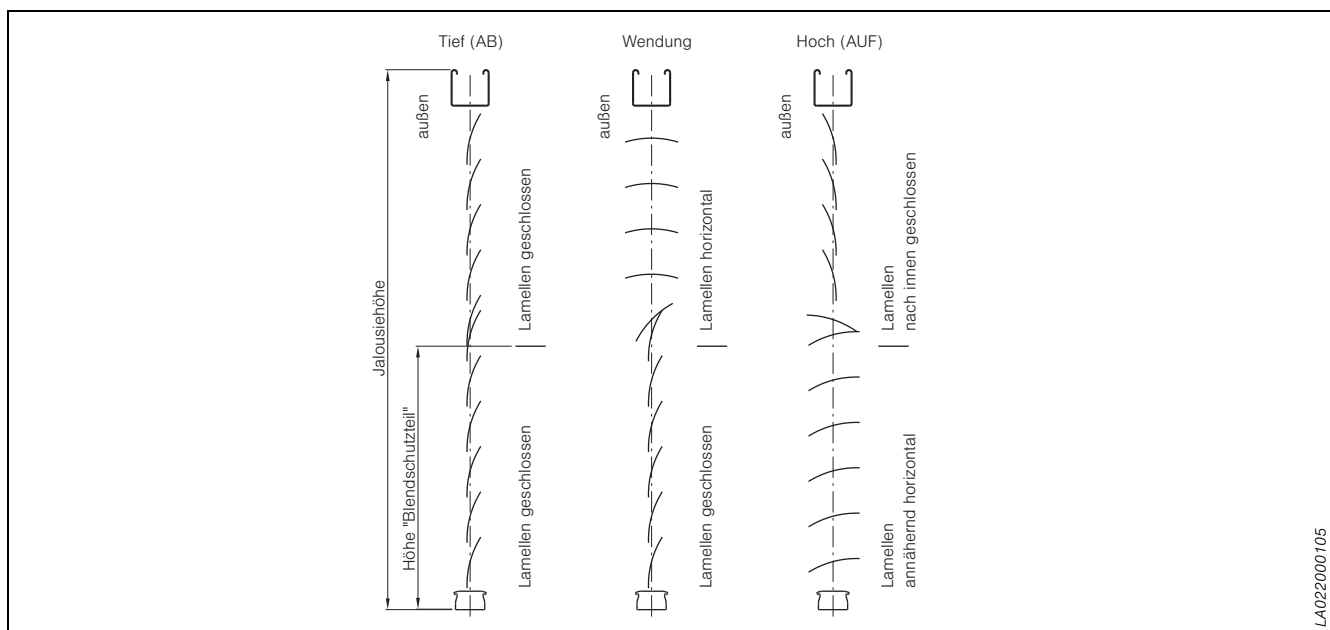
Abb. 36: Jalousie Select S mit geteilten Behängen (Tageslichttechnik)
