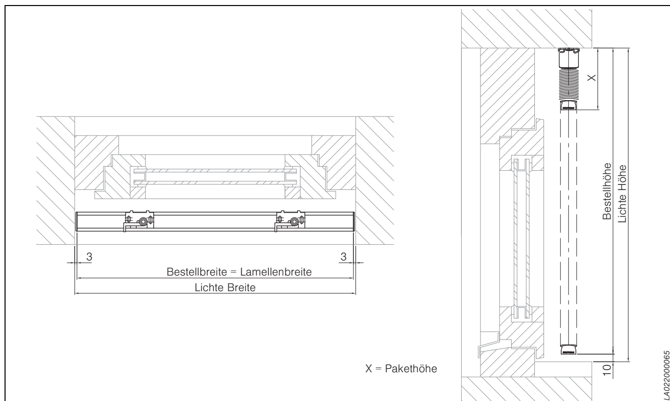
Abb. 45: Horizontal- und Vertikalschnitt – Montage in der Laibung (Einbau Pfosten-Riegel-Konstruktion)
