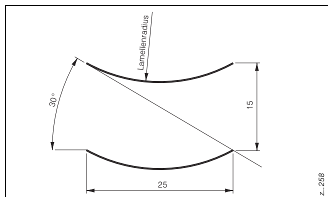
Abb. 35: Geometrie der 30°-Lichtlenklamellen
