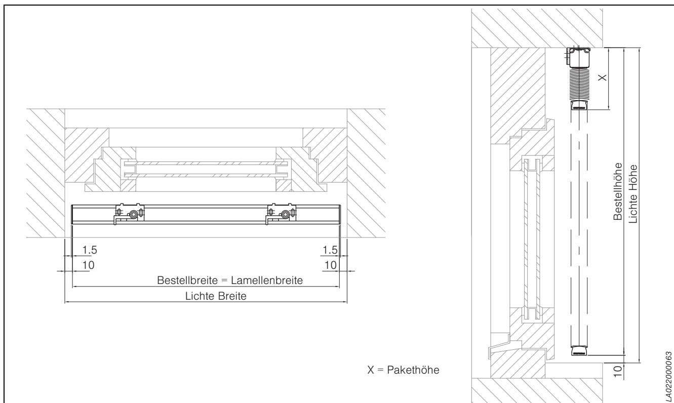
Abb. 43: Horizontal- und Vertikalschnitt – Montage in der Laibung (Einbau Mauerwerk)
