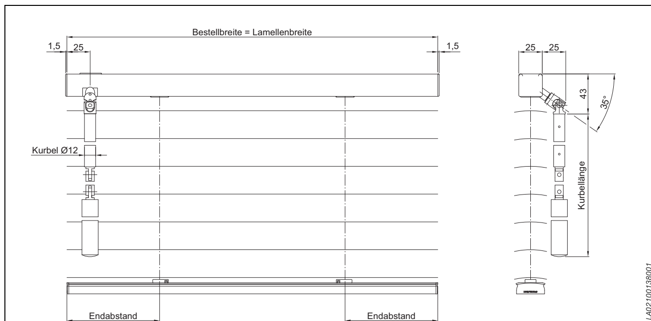
Abb. 40: Jalousie Select S – Maßanleitung, Bedienung Kurbel, Getriebeabgang stirnseitig (Standard)
