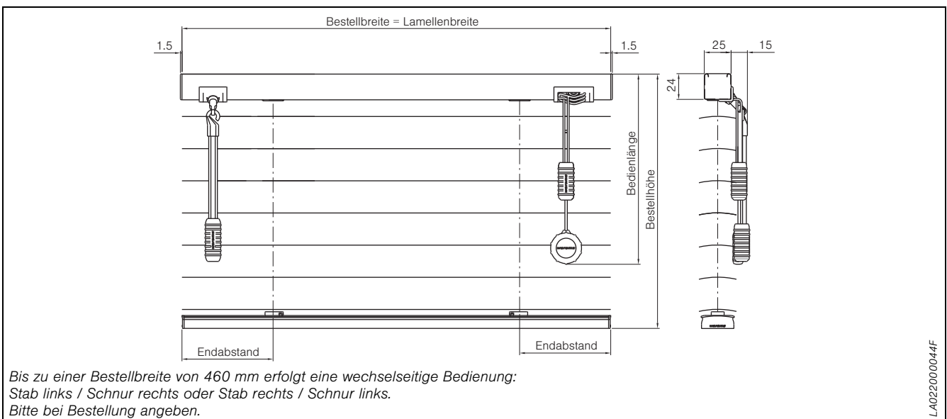
Abb. 38: Jalousie Select S – Maßanleitung, Bedienung Schnur/Stab, wechselseitig
